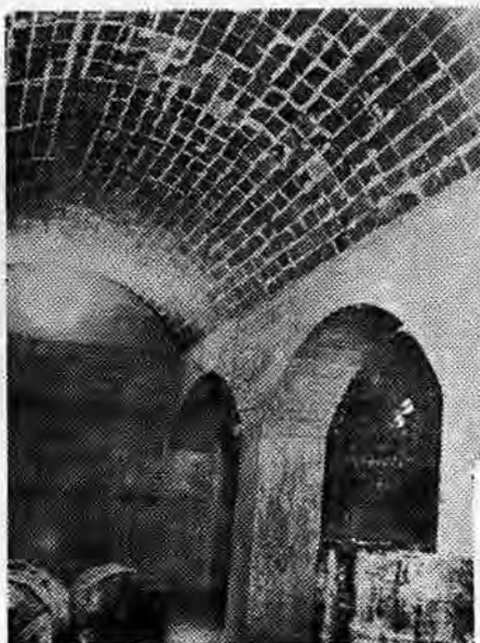
DEPOSITO DISTRIBUIDOR. —Este depósito en cola de la distribución con sus 500 metros cúbicos de capacidad asegura una dotación suficiente para las necesidades de Famoselle. En esta página puede verse ya terminado y en varias fases de su construcción. Las dos fotos interiores corresponden al detalle de una bóveda y al abovedado que cubre el depósito.
